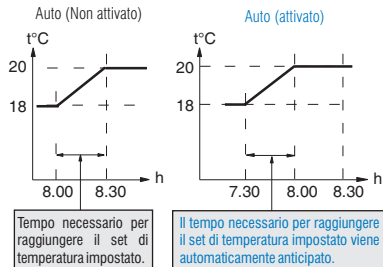
Fig. 16 Esempio in modalità inverno (riscaldamento): - accensione del cronotermostato programmata alle h 8,00 - temperatura di comfort, Set impostato 20 °C
